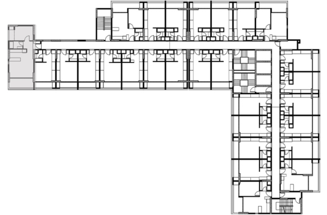
B BLOK 1.- 2.-3.-4.-5.-6.-7. KATLAR ZEMİN KAT
