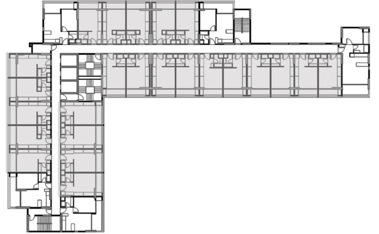
A BLOK 1.- 2.-3.-4.-5.-6.-7. KATLAR ZEMİN KAT-8. KAT
